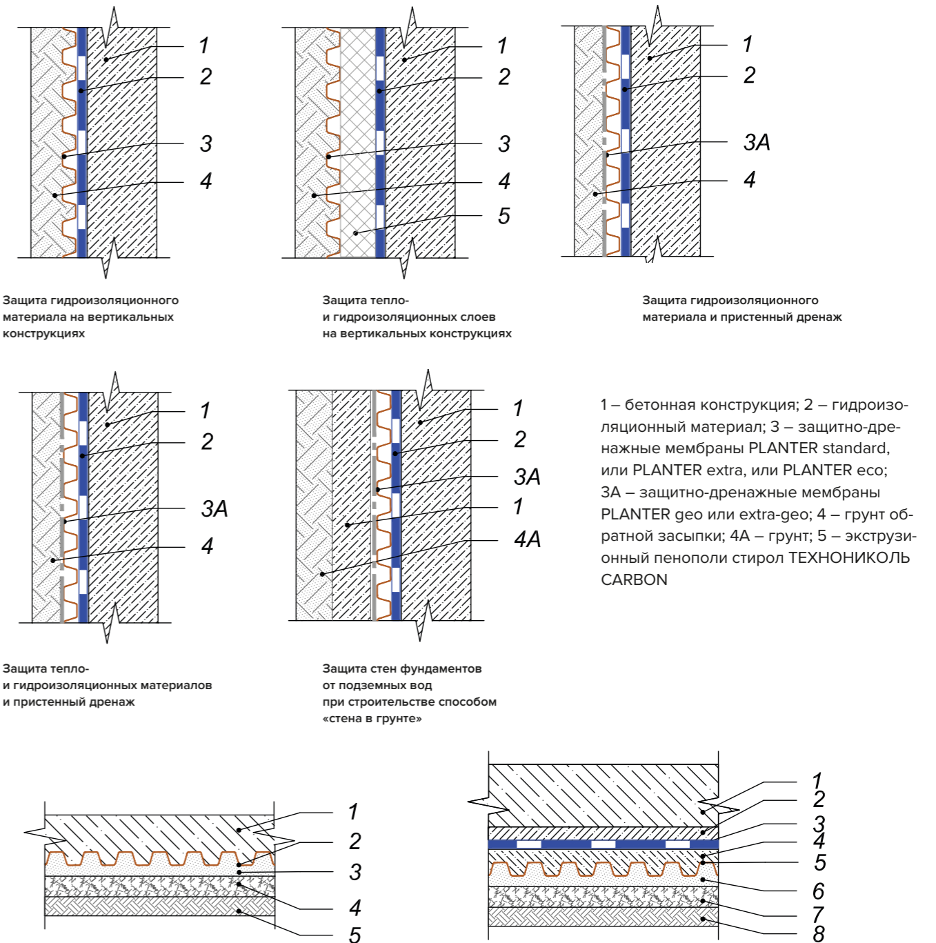
Конструкция пластового дренажа и замена бетонной подготовки
